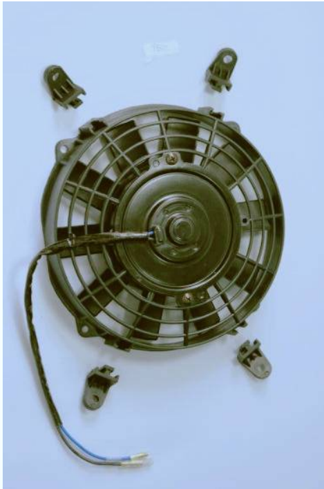
190 mm , 吸风 有刷轴流风机 12V DC Brush Axial Fan, Blowing
